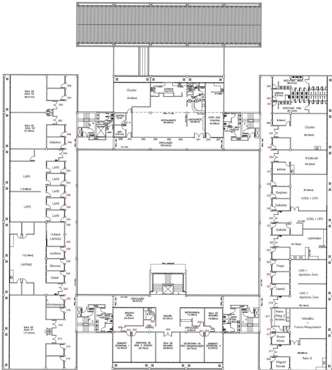
1 PLANTA 3ª PAVIMENTO ESC.: 1:100
