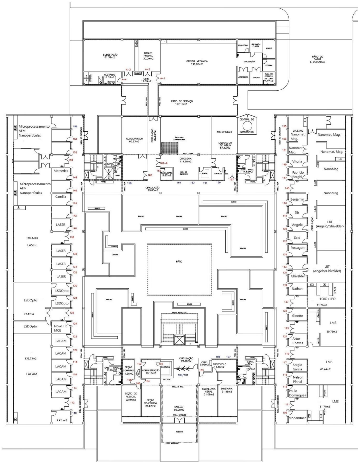
1 PLANTA 1º PAVIMENTO ESC.: 1:200
